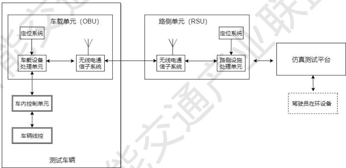
图4.1 系统组成
